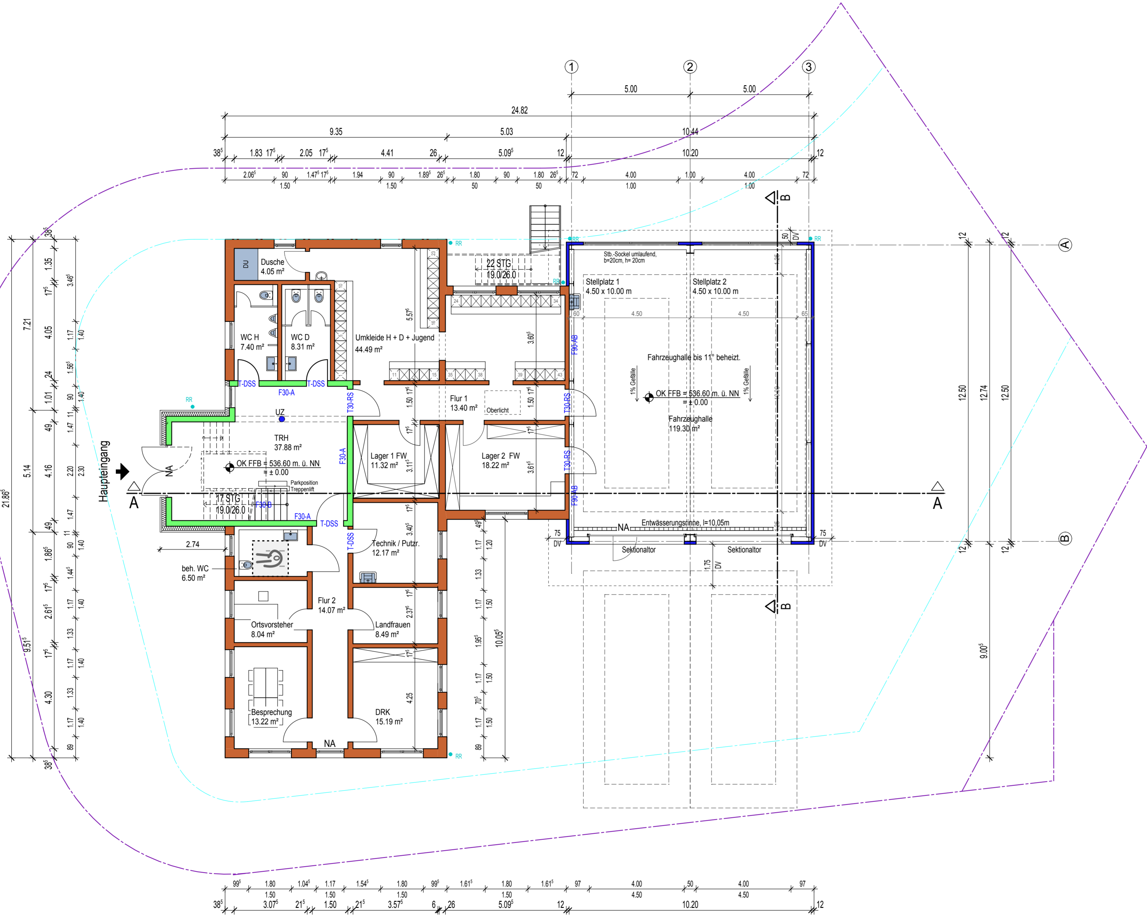
Grundriss Erdgeschoss
